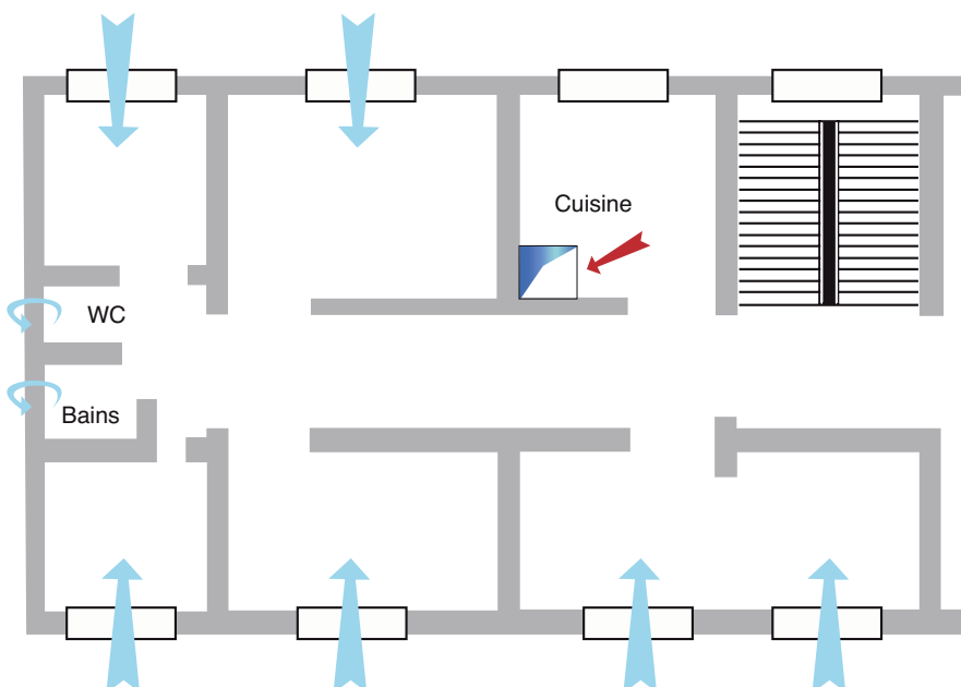
Figure 3.4 : ventilation partielle
